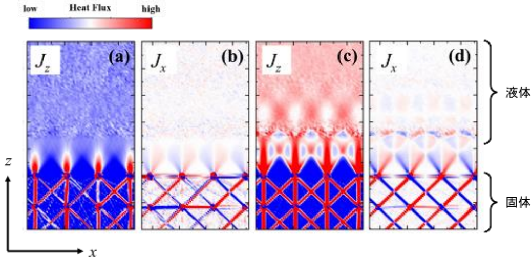
図1 固体-液体界面における2次元熱流構造( z :巨視的な温度勾配方向)。(a, b) 濡れ性が悪い場合。(c, d) 濡れ性が良い場合。 J_x と J_z はそれぞれ x 方向と z 方向の熱流束を示している。濡れ性が良い場合に顕著な熱流が観測されていることが分かる。(論文とは異なる計算条件)
