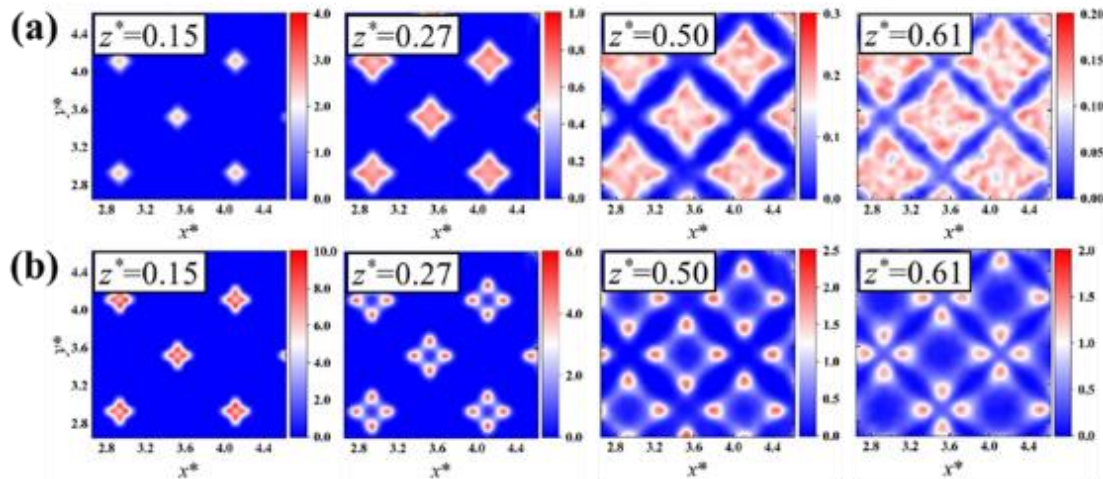
図2 固液界面内における3次元熱流構造(各 z 方向高さにおける断面で表示)。(a) 濡れ性が悪い場合。(b) 濡れ性が良い場合。濡れ性が良い場合に指向性を有する顕著な熱流が観測されていることが分かる
